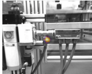
압축공기 누설에 대한 음향 이미지와 열화상 이미지 측정
