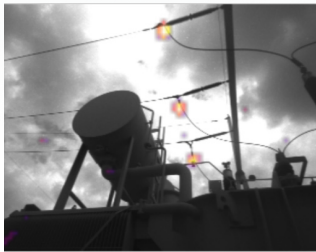
고압전선 송전선 유지 보수 (다발성 부분방전)
